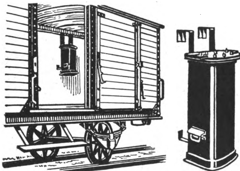
Dewag-Heizapparat im Waggon aufgehängt.
