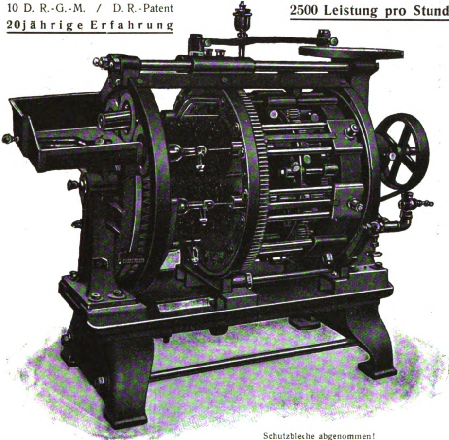
Schutzbleche abgenommen!
